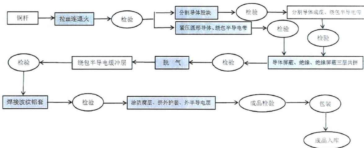
图3-1 生产工艺流程图
