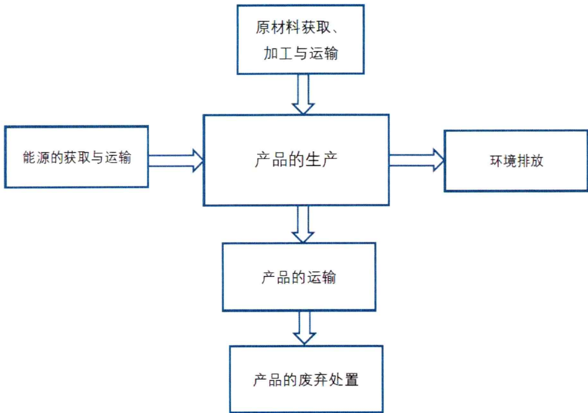
图3-2 1米额定电压127/220kV交联聚乙烯绝缘电力电缆（ZRA-YJLW02-127/220kV 1×2500）产品CFP研究边界
